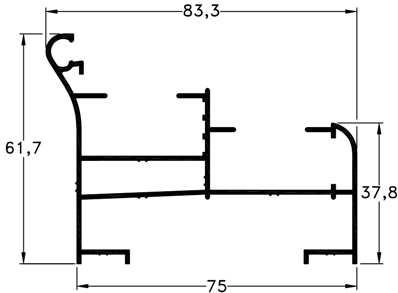
505 - Marco Ventana Guillotina peso: 0,97 Kg/m
