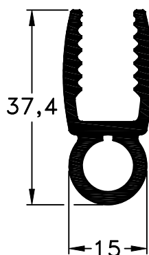
203 - Hoja peso: 0,64 Kg/m
