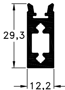
202 - Porta Hoja peso: 0,57 Kg/m
