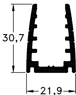
201 - Marco peso: 0,52 Kg/m
