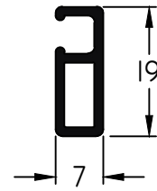
61 - Mosquitero peso: 0,17 Kg/m
