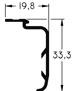
709 - Contramarco Largo Std.: 6150 mm Peso: 0,19 Kg/m
