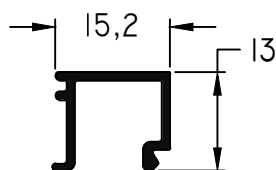
34 - Contravidrio peso: 0,14 Kg/m
