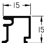
908 - Contravidrio peso: 0,16 Kg/m
