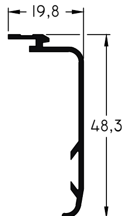
723 - Contramarco Largo Std.: 6150 mm Peso: 0,26 Kg/m
