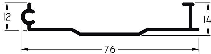
122 - Tapacinta Movil peso: 0,29 Kg/m
