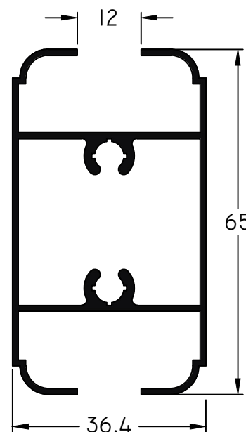
552 - Travesaño peso: 0,86 Kg/m
