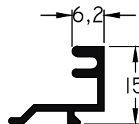
909 - Contravidrio peso: 0,16 Kg/m
