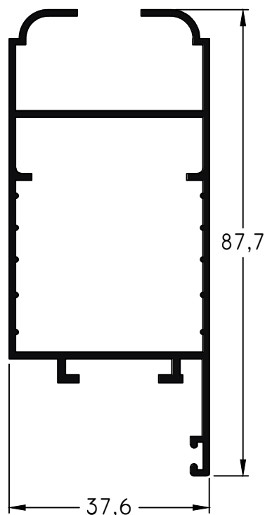
514 - Hoja Largo Std: 6150 mm peso: 0,91 Kg/m
