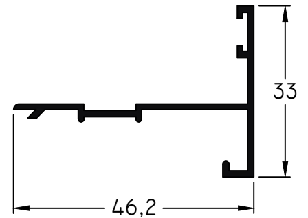
16 - Batiante Largo Std.: 6150 mm peso: 0,31 Kg/m
