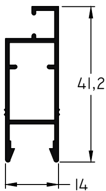
105 - Mosquitero peso: 0,32 Kg/m
