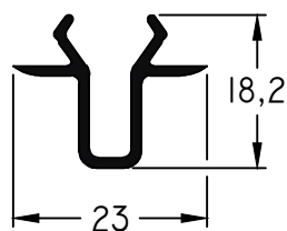
27 - Encuentro para 4 Hojas Perfil 481 peso: 0,18 Kg/m
