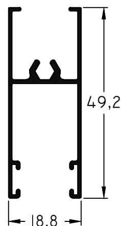
902 - Zócalo VC peso: 0,40 Kg/m
