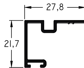
22 - Porta Felpa Zócalo peso: 0,23 Kg/m
