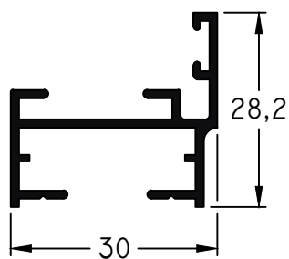
291 - Marco peso: 0,35 Kg/m
