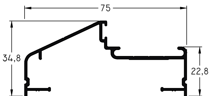
271 - Marco Largo Std.: 6150 mm peso: 0,54 Kg/m
