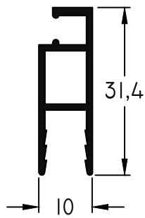
60 - Mosquitero peso: 0,25 Kg/m
