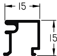
908 - Contravidrio peso: 0,16 Kg/m
