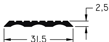
66 - Tapacanto peso: 0,15 Kg/m
