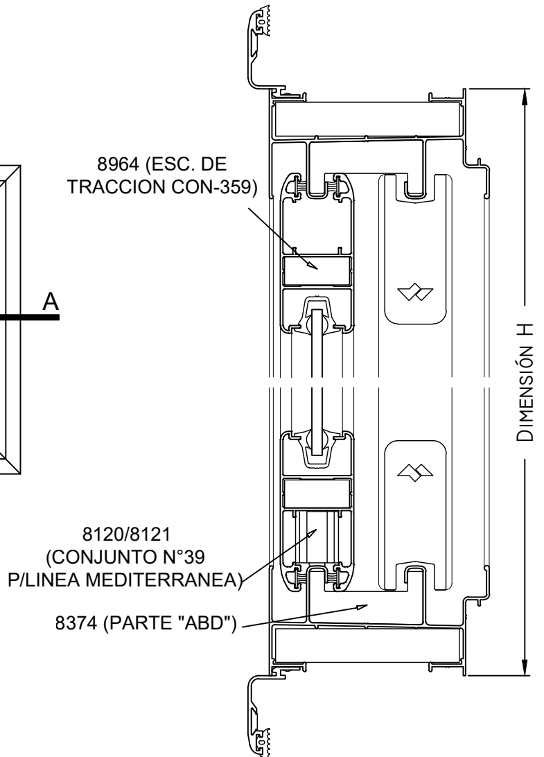
B-B Corte Vertical
