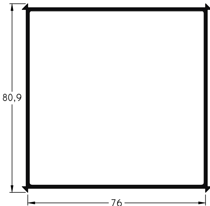
455 - Perfil Columna peso: 1,18 Kg/m
