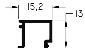
34 - Contravidrio peso: 0,14 Kg/m
