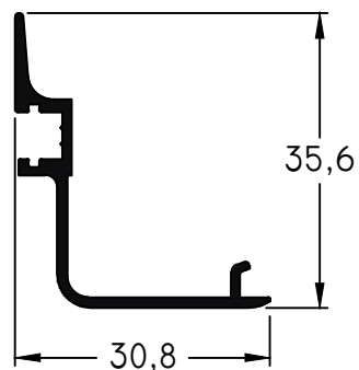
26 - Encuentro Hoja v/p Corrediza peso: 0,27 Kg/m
