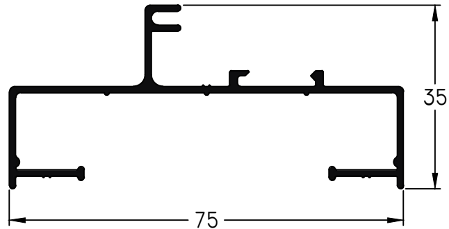
907 - Marco de Paño Fijo peso: 0,59 Kg/m
