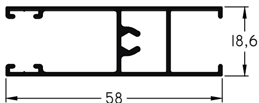
23 - Zócalo y Cabezal Ventana Corrediza peso: 0,50 Kg/m
