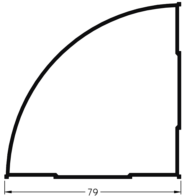
986 - Columna Curva peso: 1,06 Kg/m
