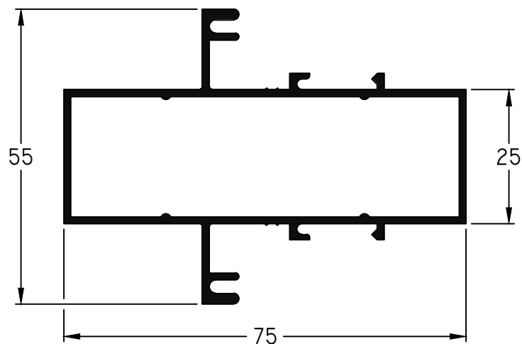
994 - Travesaño de 75 mm peso: 0,96 Kg/m
