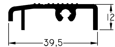
726 - Umbral Transitable peso: 0,39 Kg/m
