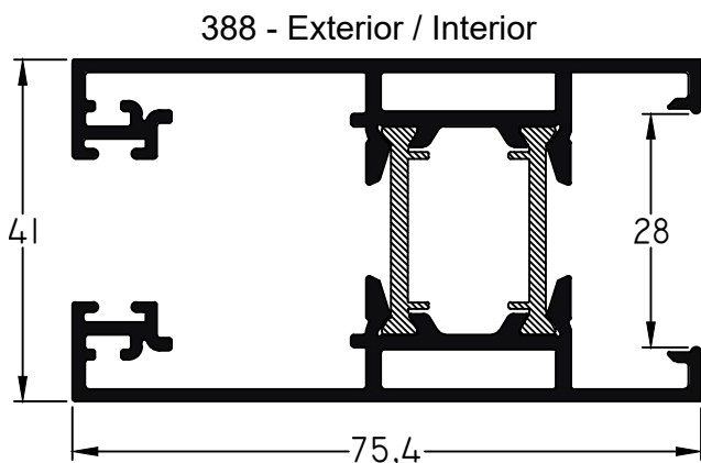
6330 - Hoja VC/PVC M-Tres RPT peso: 1,680 Kg/m
