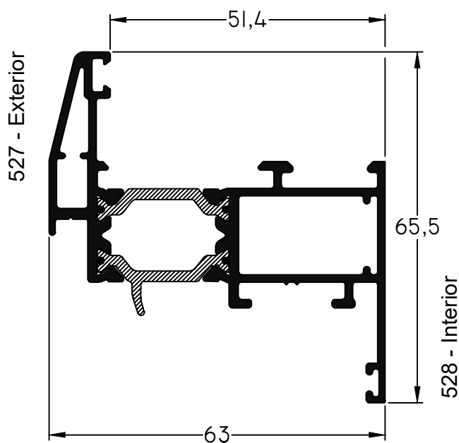
6340 - Hoja VR/VB/VOB M-Tres RPT peso: 1,32 Kg/m
