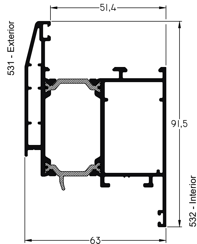
6370 - Parante Puerta M-Tres RPT peso: 1,79 Kg/m
