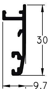
884 - Contramarco Largo std.: 6150 mm Peso: 0,20 Kg/m
