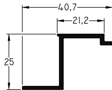
612 - Contravidrio M-Cinco de 21.2 mm peso: 0,31 Kg/m
