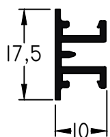
540 - Tapa Tornillo Paño Fijo M-Cinco peso: 0,15 Kg/m
