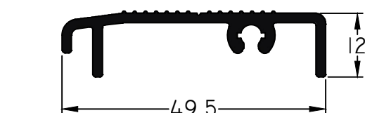
772 - Umbral Transitable M-Tres / 25mm peso: 0,44 Kg/m
