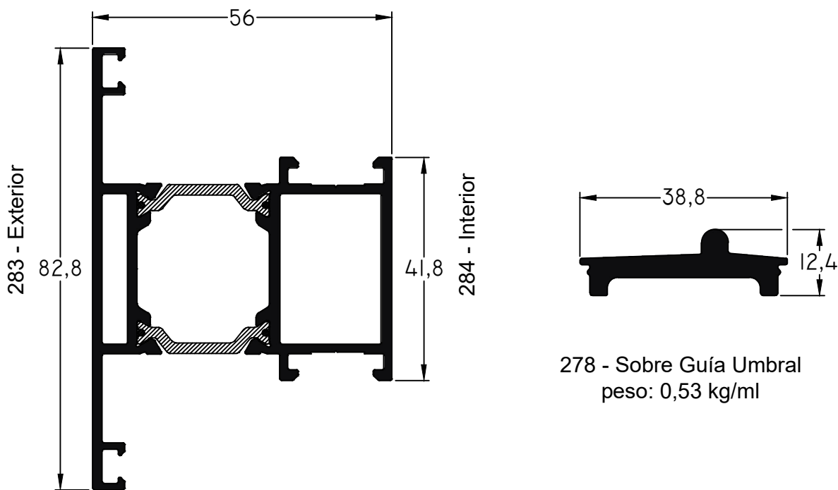
6500 - Encuentro Central Fijo-Móvil ST-MF peso: 1,62 kg/ml
