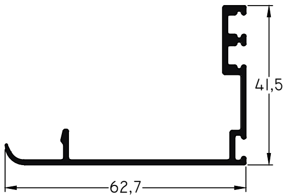
610 - Encuentro de Hoja M-Siete RPT peso: 0,50 Kg/m
