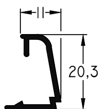
705 - Contravidrio peso: 0,16 Kg/m
