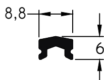
561 - Guía Inferior Corrediza peso: 0,09 Kg/m
