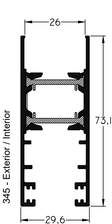
6280 - Hoja VC/PVC M-Uno RPT peso: 1,23 Kg/m
