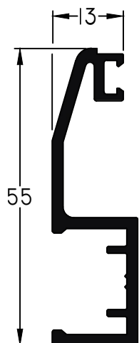
859 - Soporte Vidrio M-Cinco peso: 0,57 Kg/m
