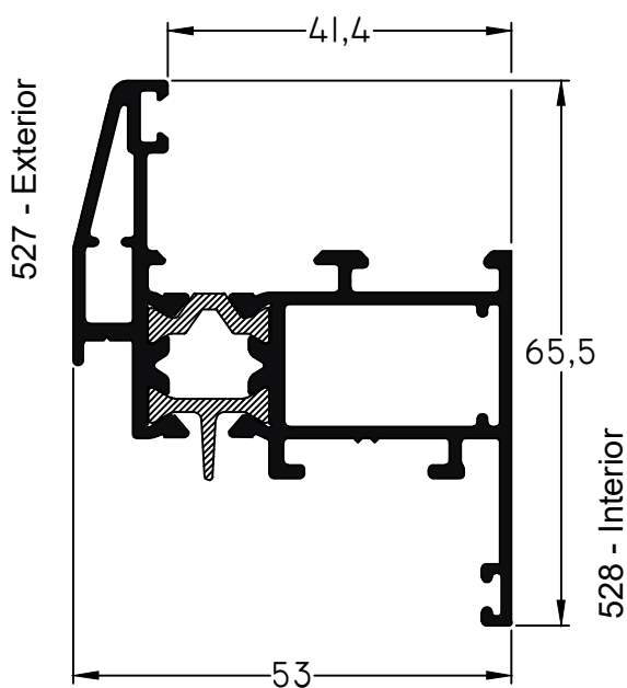
6140 - Hoja VR/VB/VOB M-Tres RPT peso: 1,26 Kg/m
