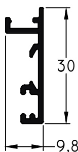
693 - Contramarco Largo Std.: 6150 mm peso: 0,20 Kg/m
