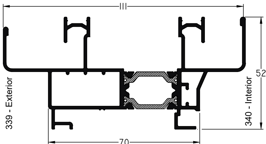
6390 - Marco VC/PC M-Tres RPT peso: 1,80 Kg/m
