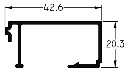
286 - Tapa Horizontal Lado Móvil peso: 0,37 kg/ml
