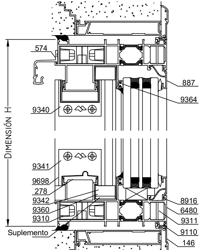
C-C Corte Vertical
