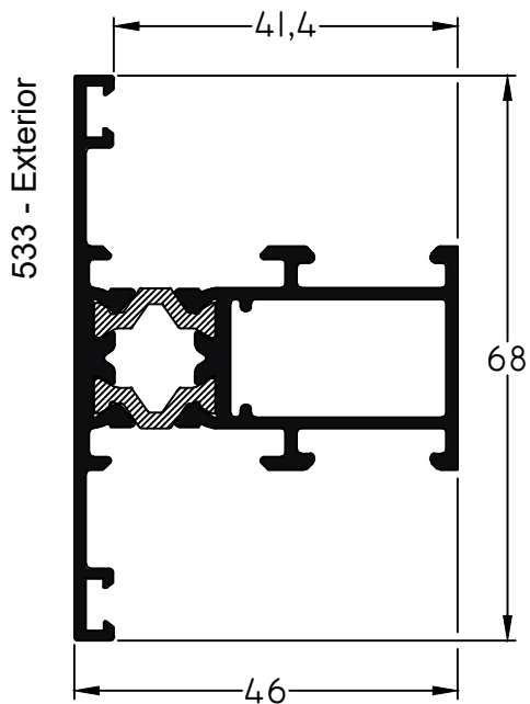
6160 - Travesaño M-Tres RPT peso: 1,17 Kg/m
