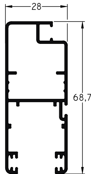
738 - Mosquitero Reforzado peso: 0,80 Kg/m
