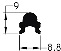
543 - Guía Inferior corrediza radio 3 mm peso: 0,13 Kg/m
