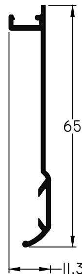
857 - Contramarco largo std.: 6150 mm peso: 0,27 g/m
