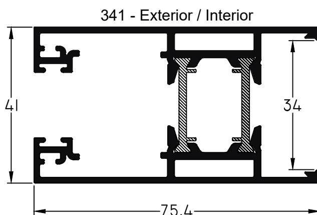
6400 - Hoja VC/PC M-Tres RPT peso: 1,65 Kg/m
