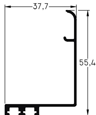
317 - Encuentro M-Cinco RPT peso: 0,38 Kg/m
