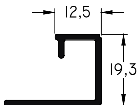
282 - Compensador Hoja peso: 0,24 kg/ml
