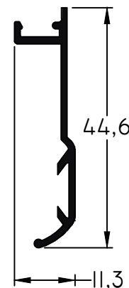
862 - Contramarco largo std.: 6150 mm peso: 0,21 Kg/m
