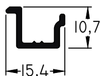
519 - Adaptador Porta-Burlete para 6350 peso: 0,11 Kg/m
