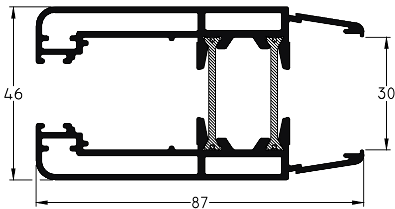
6530 - Hoja Corrediza M-Cinco RPT peso: 2,06 Kg/m
