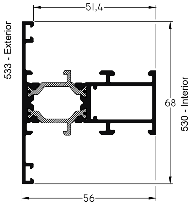
6360 - Travesaño M-Tres RPT peso: 1,20 Kg/m
