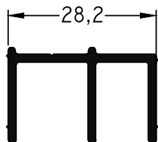
270 - Suplemento cerradero jamba peso: 0,31 kg/ml
