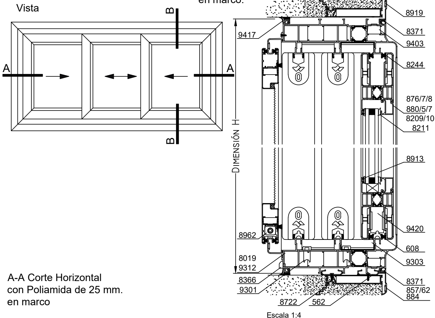
B-B Corte Vertical con Poliamida de 25 mm en marco.
