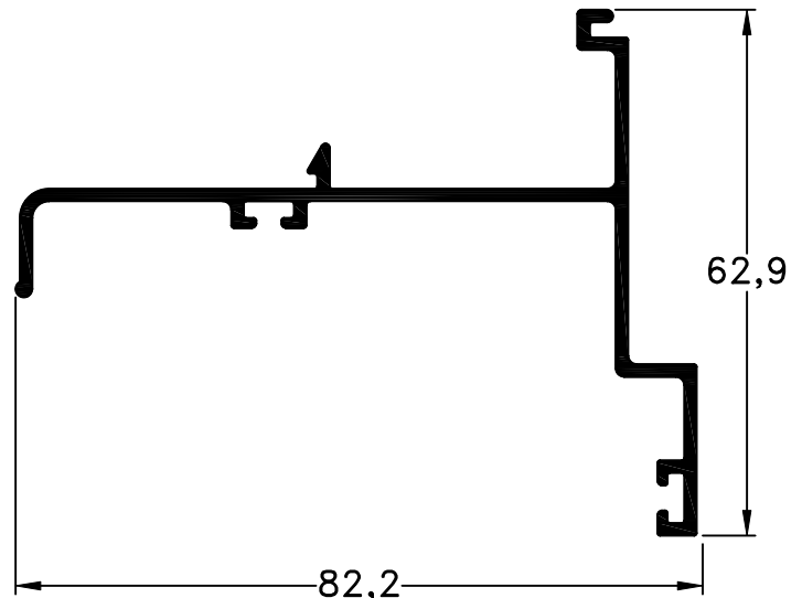
359 - Bota Agua paño de Abrir p/ V.S peso: 0,75 Kg/m
