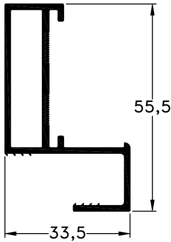
374 - Cabezal / Zócalo de Hoja p/V.S peso: 0,68 Kg/m
