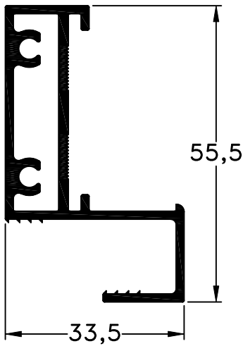
373 - Parante de Hoja p/V.S peso: 0,78 Kg/m
