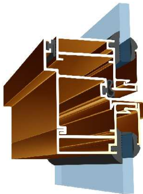
Modelo en 3D - Hoja 377 con Bota Agua 378
