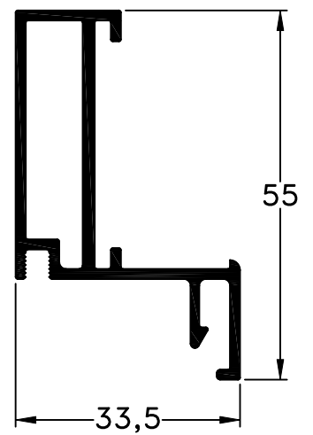
377 - Hoja c/Contravidrio p/V.S peso: 0,69 Kg/m
