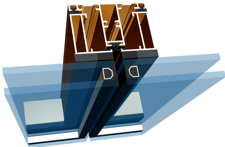
Modelo en 3D - Columna Divisoria 367 opción DVH
