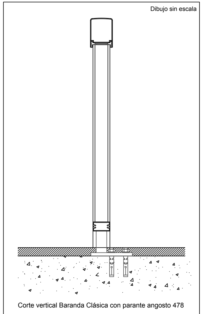
478 - Parante Angosto peso: 0,51 Kg/m
